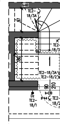
RZUT PARTERU
