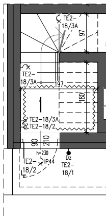
RZUT PIĘTRA
