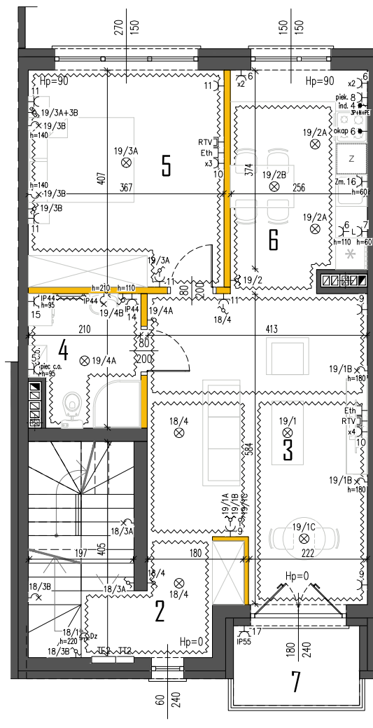
RZUT PIĘTRA
