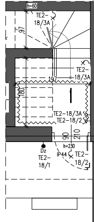
RZUT PARTERU
