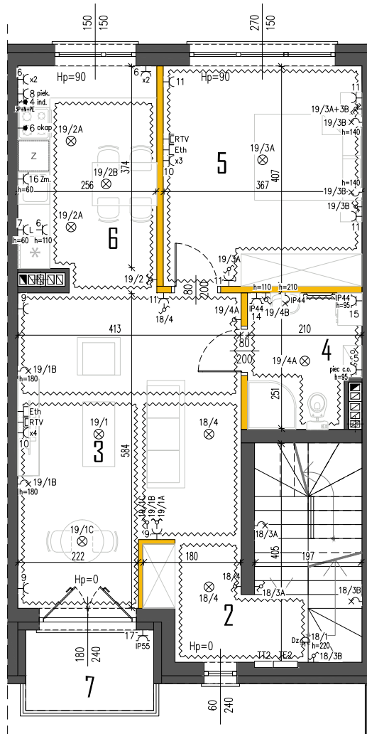
RZUT PIĘTRA
