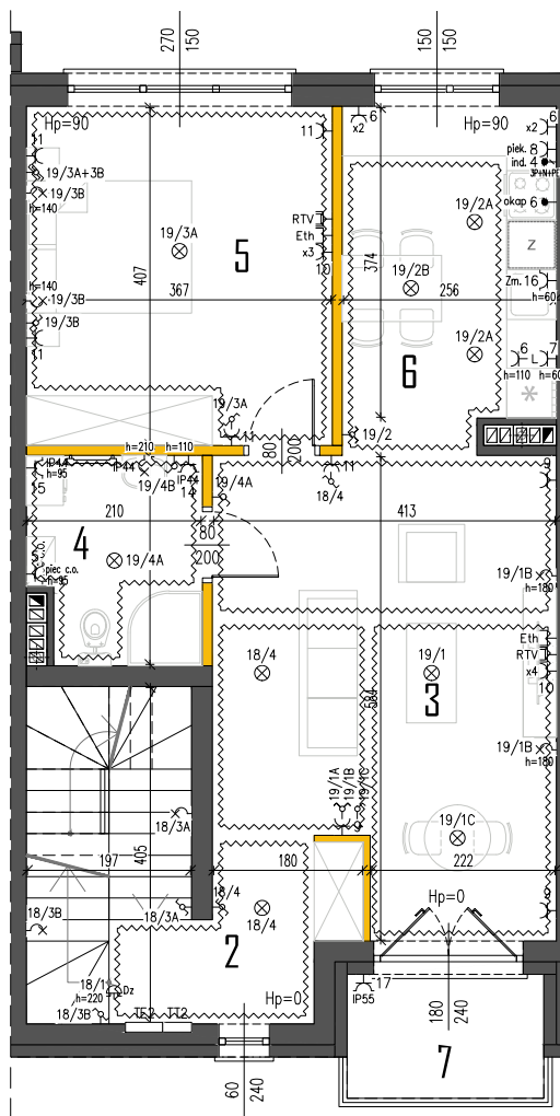
RZUT PIĘTRA
