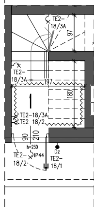
RZUT PARTERU
