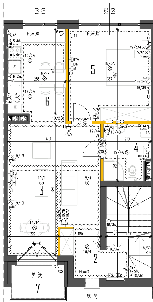
RZUT PIĘTRA
