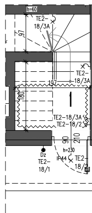
RZUT PARTERU
