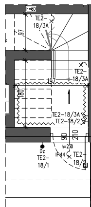
RZUT PARTERU
