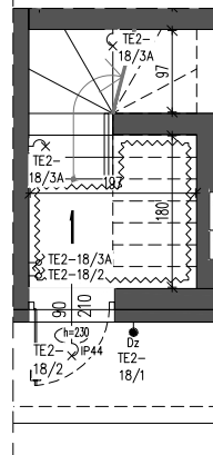
RZUT PARTERU
