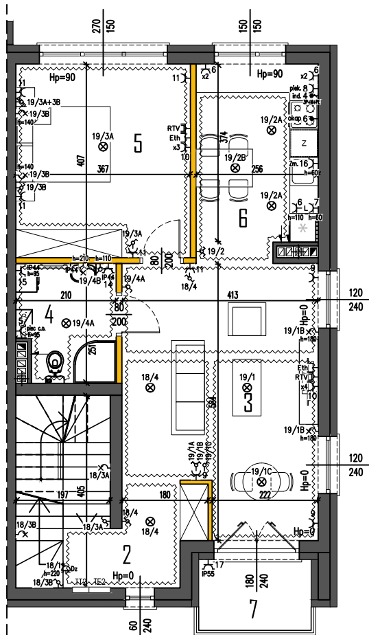
RZUT PIĘTRA
