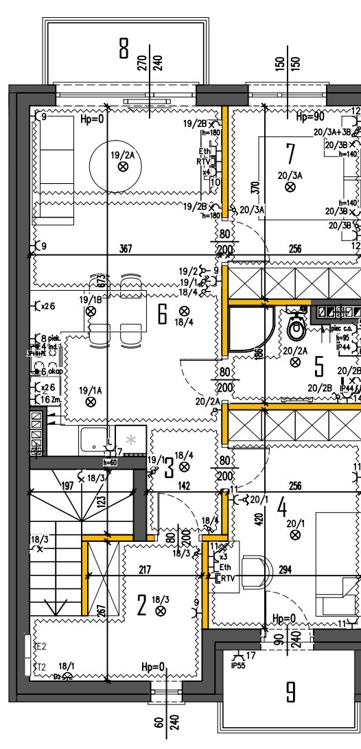
RZUT PIĘTRA
