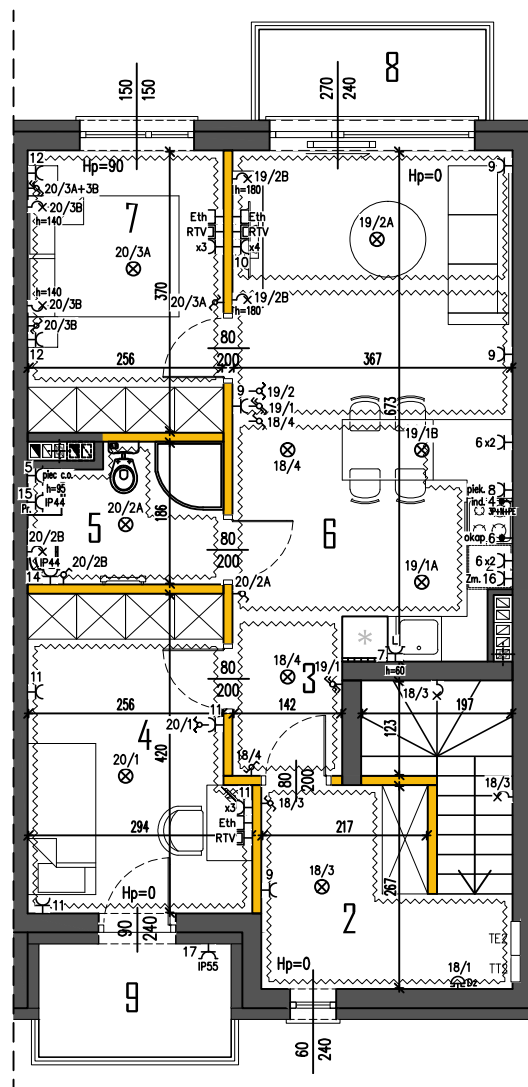
RZUT PIĘTRA
