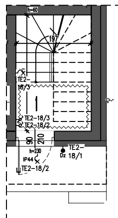
RZUT PARTERU
