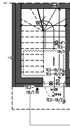
RZUT PARTERU
