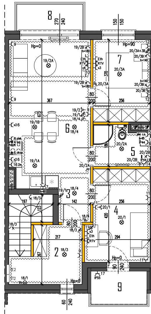
RZUT PIĘTRA
