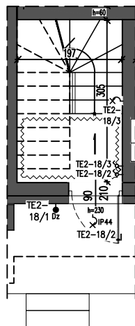
RZUT PARTERU
